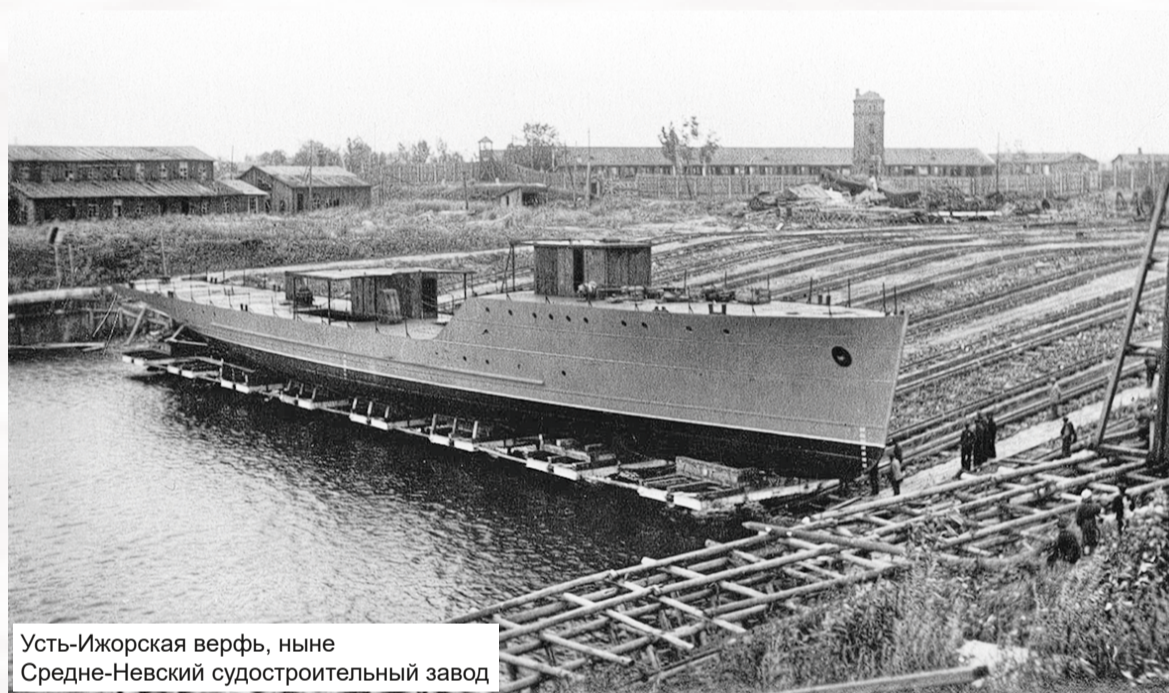
БТЩ Т-206 «Верп» – один из базовых тральщиков, построенных по проекту 53У. Фото сделано финской разведкой накануне войны
